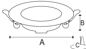
ÖLÇÜLER/ DIMENSIONS
